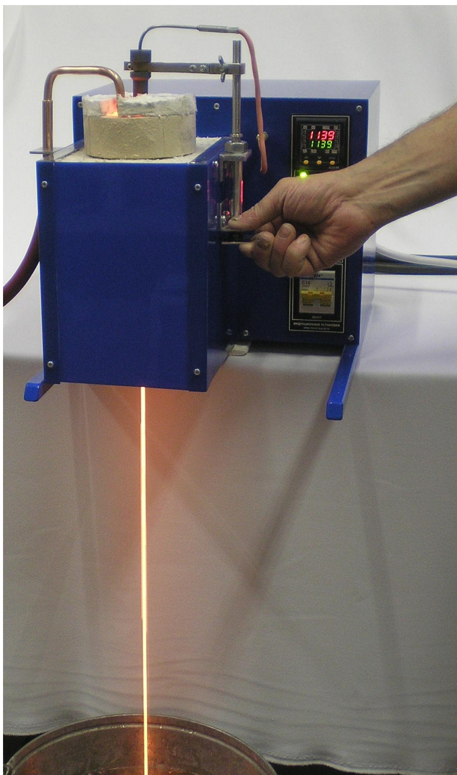
Рисунок 7 - донный розлив металла.
